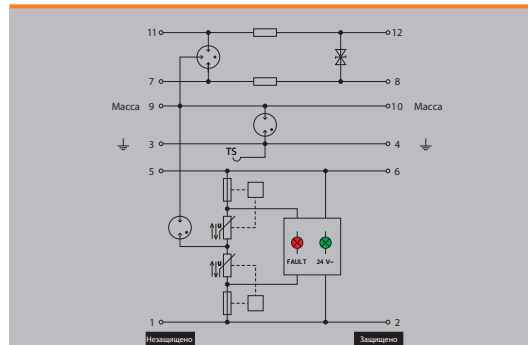
Комплектный модуль, непрямого заземления
