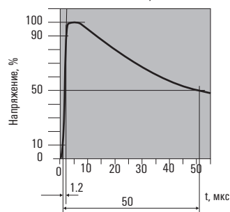
Испытательный импульс 10 / 350 мкс
