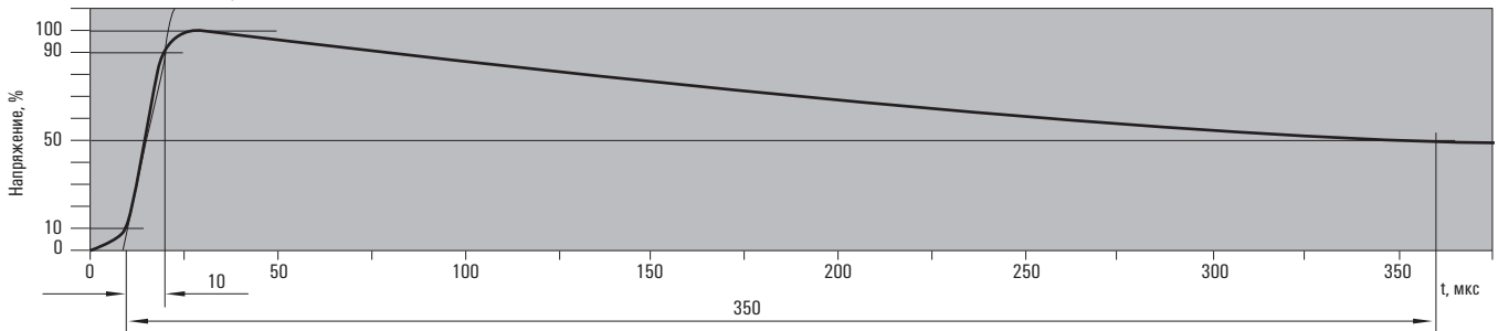
Испытательный импульс 10 / 350 мкс
