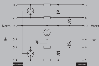
Комплектный модуль, непрямого заземления
