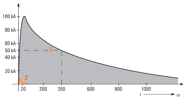
Испытательный импульс 10 / 350 мкс
