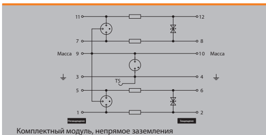
Комплектный модуль, не прямое заземления
