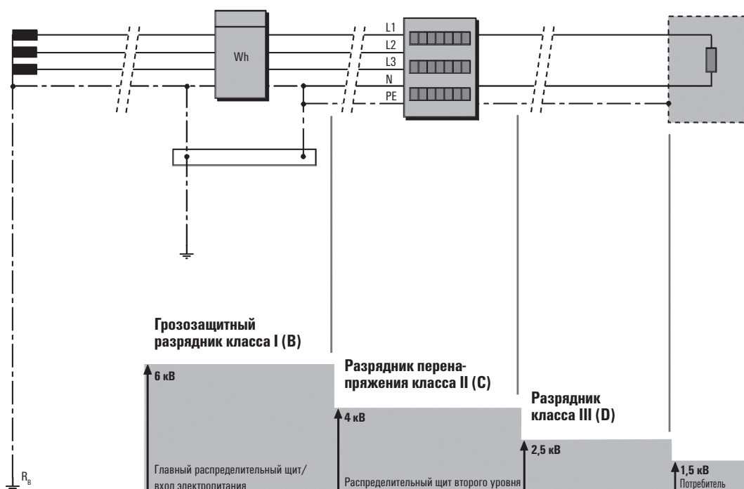
Расчетное импульсное перенапряжение при напряжении проводник-земление 300 В
