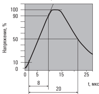
Испытательный импульс 8 / 20 мкс
