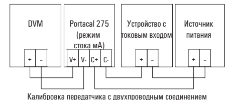
Калибровка передатчика с двухпроводным соединением
