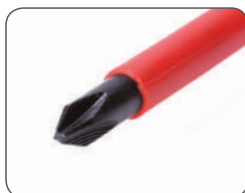
Засечки от соскальзывания на профиле «Phillips»
