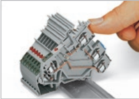
Установка на несущую рейку. Клеммы с заземлением автоматически устанавливают контакт с рейкой.
