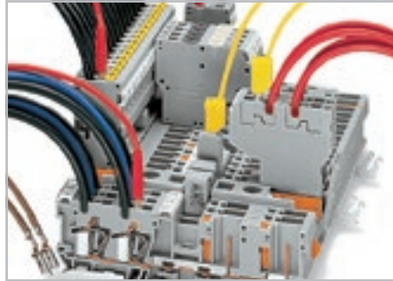
Проверка с помощью тестового штекера 2 мм Ø (красный) или 2,3 мм Ø (желтый).
