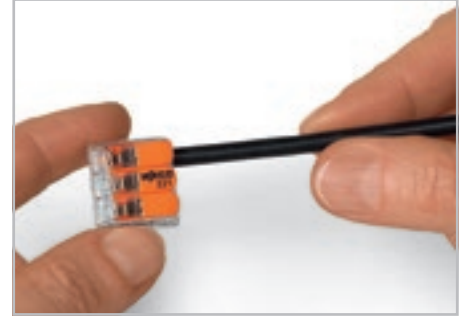
Затем опустите рычаг, чтобы замкнуть зажим.
