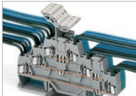
Объединение вертикальными и поперечными перемычками.
