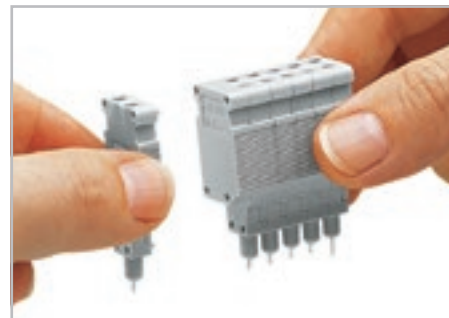
Соединение тестового штекера и модулей разделителей для сборки многоконтактного модуля тестового штекера (максимум 10 контактов).
