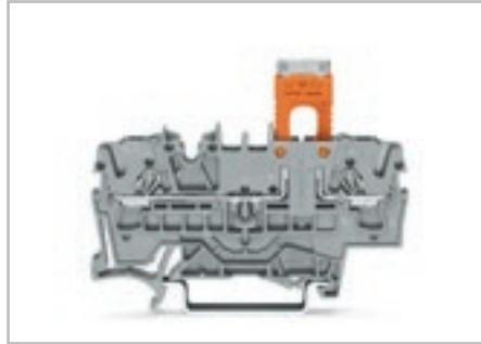
Базовая клемма с размыкателем в исходном положении. На примере применения показана 2-проводная базовая клемма 2002-1661 с разъединителем
