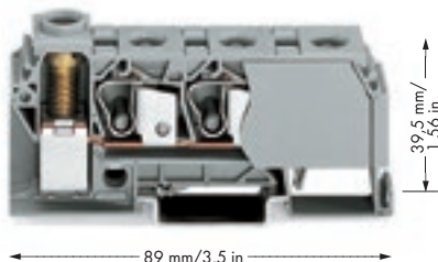
Заделка проводника 35 мм 2 /AWG 2. Соединительный винтовой зажим, ввод проводника сбоку.
