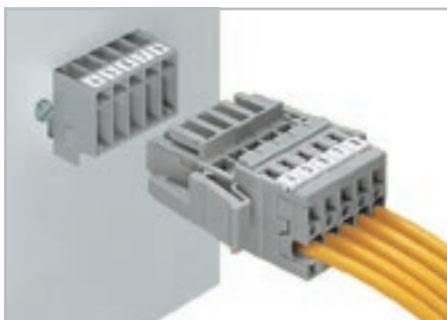
Штекер с крепежными фланцами 1-проводная розетка с боковым фиксирующим рычагом
