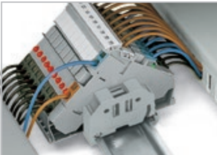
Клеммы для датчиков. Подвод питания со стороны шкафа управления.
