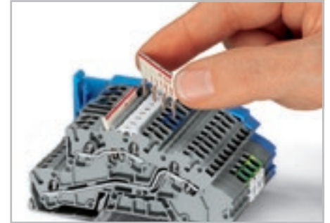
Вставьте перемычку «через один» Утопите перемычку до упора.
