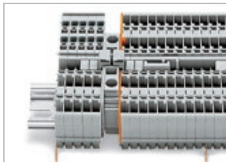
Ступенчатые перемычки используются для объединения клемм различных размеров (макс. 10 мм²/AWG 8).
