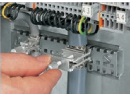
Затяжка/удаление зажима для экрана.
