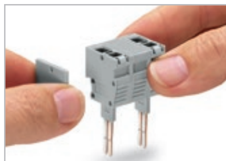
Соединение тестового штекера и модулей разделителей с разделительной пластиной для сборки многоконтактного модуля тестового штекера (макс. 10 контактов) для клеммы шириной 10 мм.
