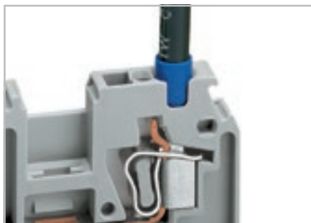
Использование кабеля AWG 12 с наконечником (Код 216-206)
