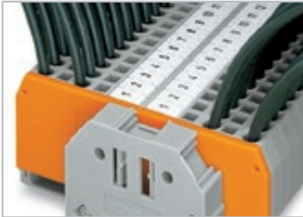
Система WMB позволяет маркировать сами клеммы. Информация по мультимаркировочной системе WMB находится в разделе 13.
