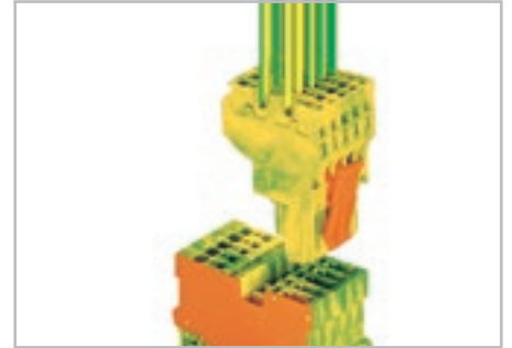
1-проводная/1-контактная базовая клемма с заземлением 2-проводная розетка, желто-зеленая
