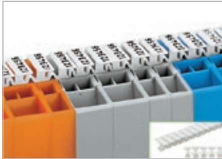
Т-образная маркировочная бирка (код 209-290)
