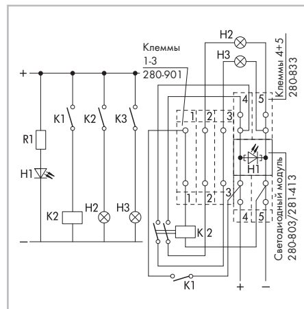
Устройство управления
