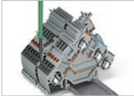
Демонтаж с несущей рейки. Внимание: предварительно снимите перемычки.
