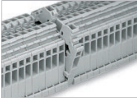
Ключи для быстрого монтажа предотвращают перевернутый монтаж.
