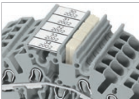
Смежные перемычки для непрерывного объединения
