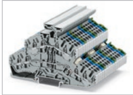
Двухуровневые клемм
