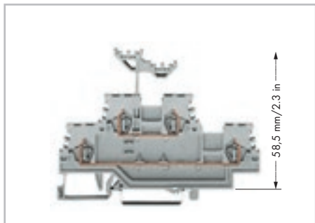
Двухуровневый держатель для маркировки Высота включает двухуровневый держатель для маркировки WSB
