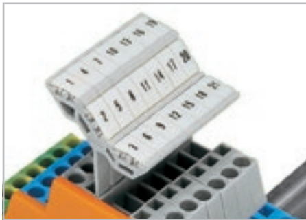
Маркировка мультимаркировочной системой WMB. Другие системы см. в разделе 13.
