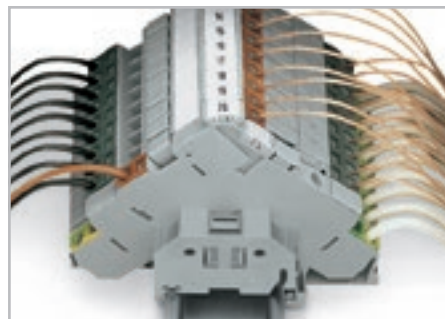
Желто-зеленый зажим = экранированный контакт
