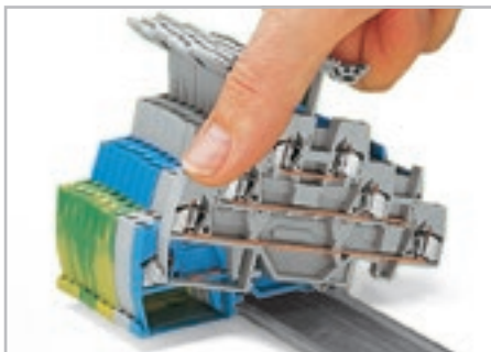
Закрепление клеммы на несущей рейке.
