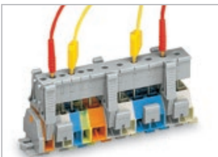
Для измерения модули тестового штекера устанавливаются в клеммную колодку – с проводом или без. Как только произошел контакт с элементом CAGE CLAMP® (нержавеющая сталь), данный тип будет ограничен до 0,5 А.
