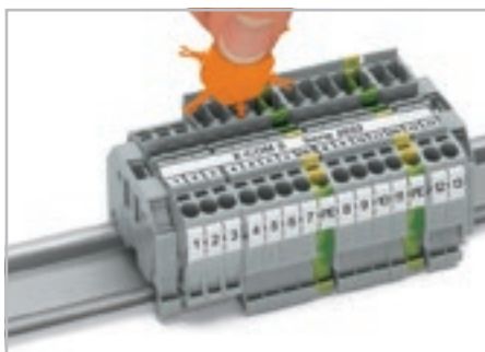
Вставьте кодирующий штифт в соответствующий разъем и отломите его.
