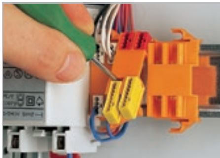
Извлечение клемм PUSH WIRE® из держателя.
