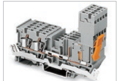
Розетка, закрепленная блокирующими рычагами в наружной части несущей клеммы.
