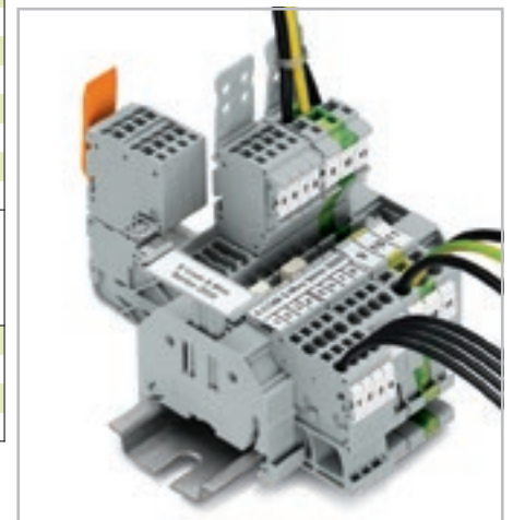
Клемная колодка X-COM®S-SYSTEM
