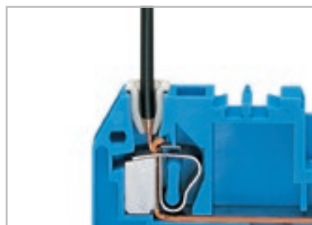
Упор-ограничитель позволяет избежать попадания изоляции проводника в зажим.
