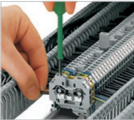
Зажим проводника
