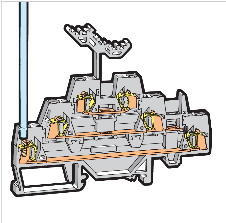
Объединение поперечными перемычками 280-402. Утопите поперечную перемычку до упора.
