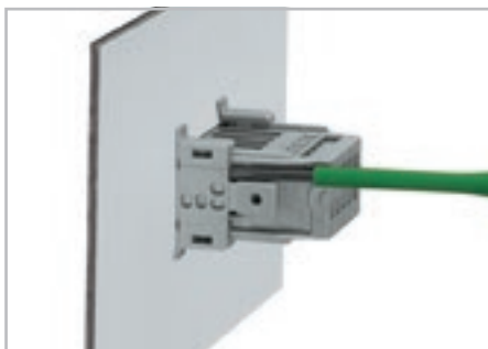
Для отсоединения вставьте рабочий инструмент (ширина лезвия 2,5 мм) в разблокирующий разъем.
