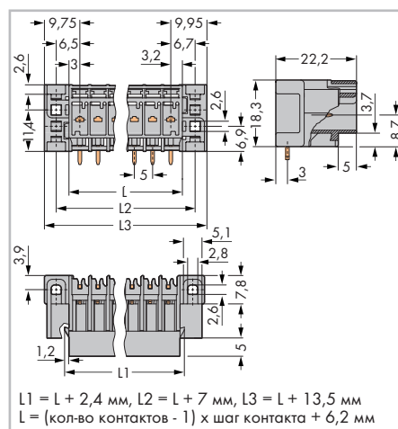
Штекер и 1-проводная розетка с поперечными фиксирующими рычагами.
