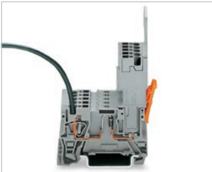
1-проводная розетка Перемычки не устанавливаются в диодные клеммы.
