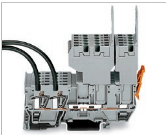
1-проводная розетка и 2-проводная розетка Объединение базовых клемм возможно только с помощью поперечных перемычек и перемычек "через один" серии 280.
