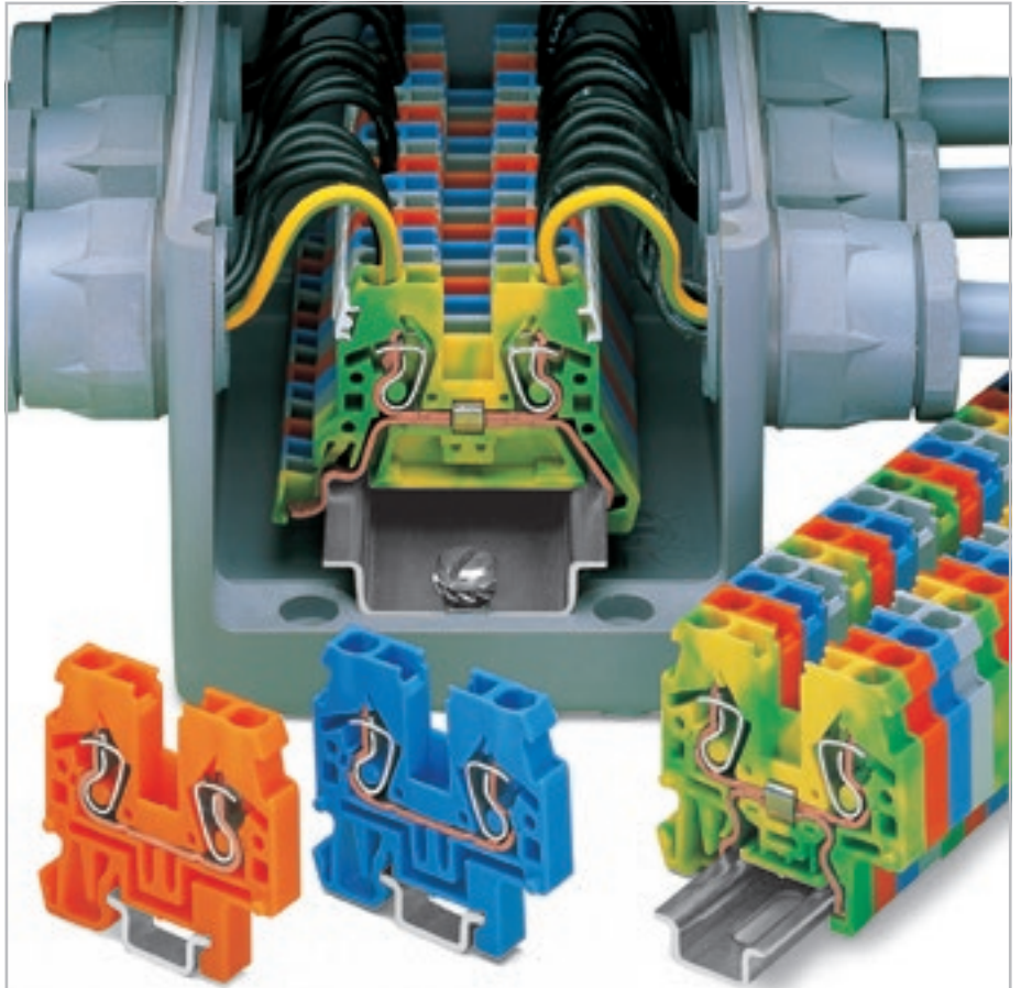
Две перемычки параллельно размещаются в клемме.
