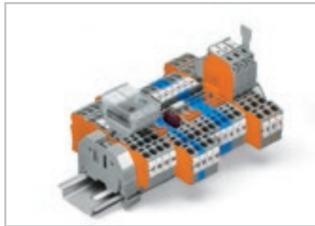
Диодный модуль установлен в проходную клемму.
