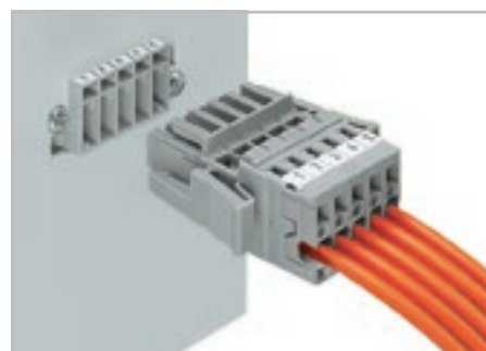
Вилка и 1-проводная розетка с боковым фиксирующим рычагом
