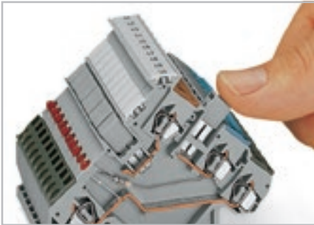
Объединение вертикальными поперечными перемычками. Утопите поперечную перемычку до упора.
