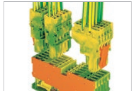
4-контактная базовая клемма с заземлением 1-проводная розетка, прямая 2-проводная розетка
