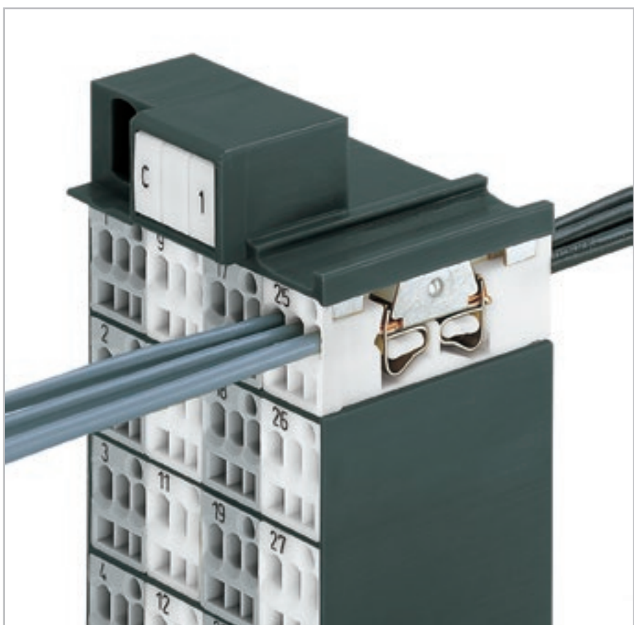
Крепление на защелке дополнительного модуля с контактом к монтажному каркасу.
