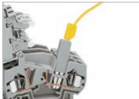
Контроль напряжения на входе при помощи тестового адаптера 280-404 (показан на рисунке) или тестового штекера 281-407.
