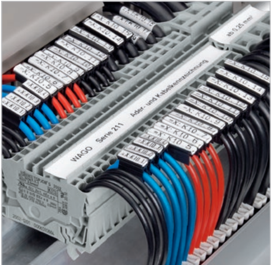
Вставьте маркер для принтера в паз для маркировочного манжеты. Замена маркера возможна и после подключения проводника.
