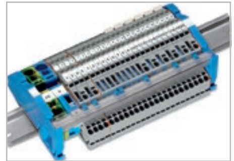
Дополнительная прозрачная крышка распределительной шины (777-303) предохраняет шину от непреднамеренного контакта и позволяет легко проверить подключенные к шине клеммы.
