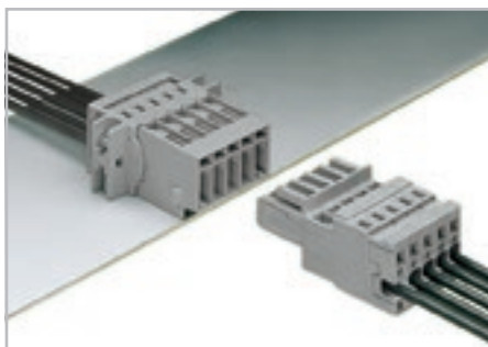
Вилка с соединением CAGE CLAMP® и фиксирующими фланцами 1-проводная розетка, прямая
