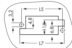
Штекер-розетка с боковым фиксирующим рычагом
