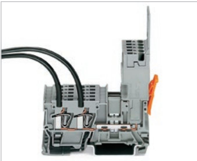
1-проводная розетка Объединение базовых клемм с помощью перемычек серии 280 и 780, проверка с помощью тестового адаптера 280-4...
