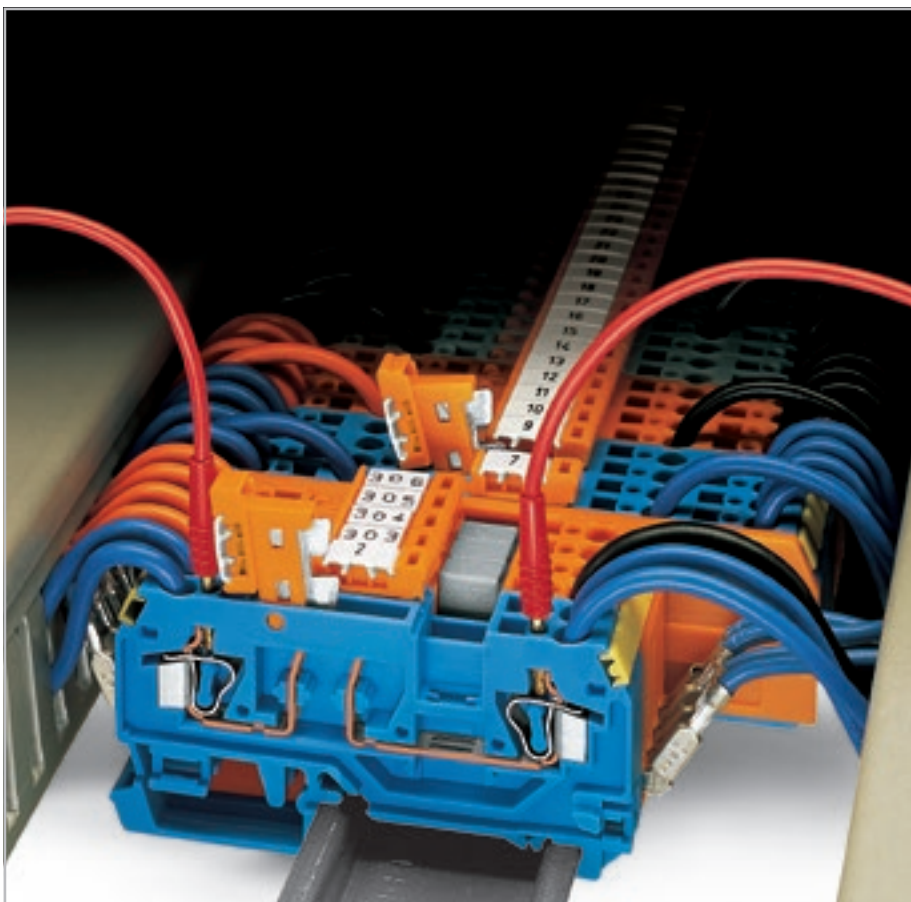
Распределение мощности с использованием ножевого разъединителя, отключение всех выходов.
