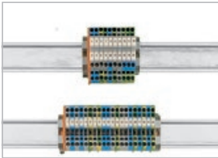
Сохраните 50% пространства рельса, используя двухуровневые клеммы.
