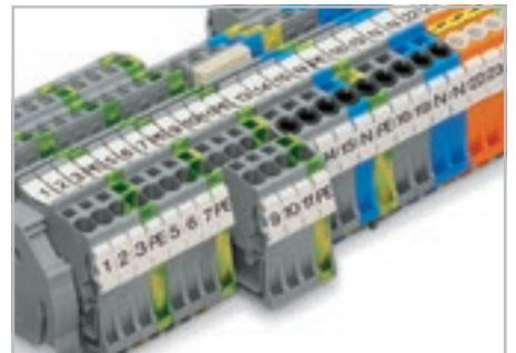
Маркировочная полоска для центральной маркировки
