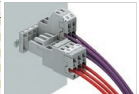
Штекер и 1- и 2-проводные розетки
