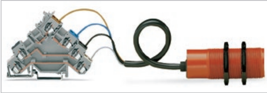
Клемма для датчика с 4-проводным датчиком
