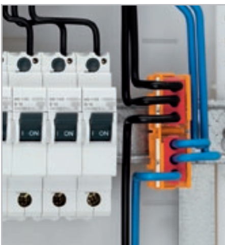
Подключение одножильных и многожильных проводников 6 мм 2 /AWG 10.
