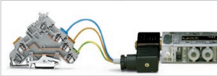
Клемма для исполнительного устройства, спаренная с электромагнитным клапаном с заземлением
