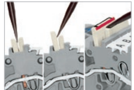
Снятие перемычки «через один» Вставьте рабочий инструмент между перемычками и поднимите перемычку.
