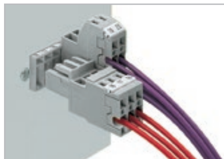
Штекеры с прямыми или угловыми контактами под пайку и проходными фланцами 1-проводная розетка, прямая 2-проводная розетка
