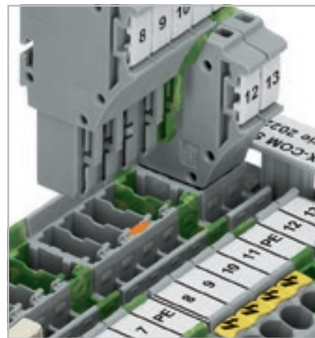
Вставьте кодирующий штифт 2022-100 в соответствующее место базовой клеммы.
