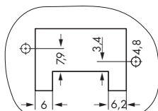
Отверстия для фиксирующих рычагов с одним контактом
