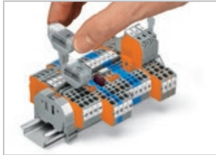
Установка диодного модуля в проходную клемму.
