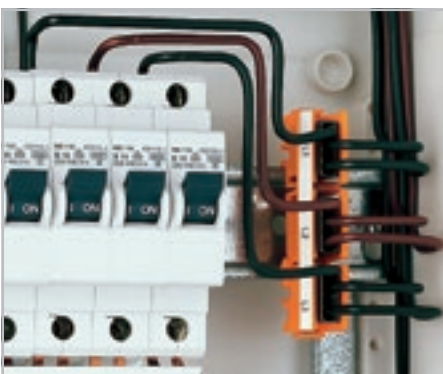
ЗАФИКСИРОВАННОЕ ПОЛОЖЕНИЕ – на DIN-рейке 35 мм
