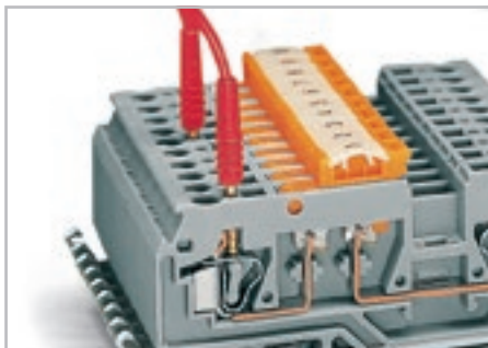
Тестовый разъем: для тестовой штекера 2 мм Ø или 2,3 мм Ø – с прямым подключением к токопроводящей шине.
