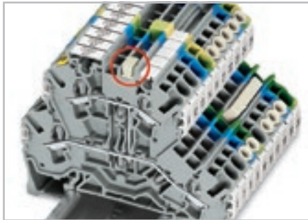
Двухуровневая вертикальная перемычка, установленная.
