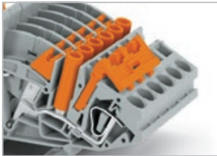
Перемычка с предохранительным колпачком Продольные переключаемые клеммы с размыкателем с установленной перемычкой, включая предохранительный колпачок
