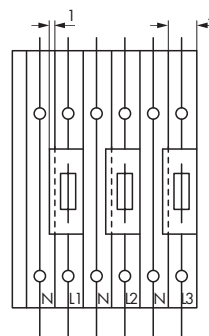
Открытая сторона клеммы. вид слева
