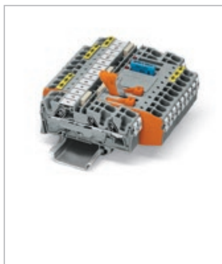
Комплект клемм включает: Проходные клеммы Разъединительные клеммы N-проводников Клеммы для автомобильных предохранителей
