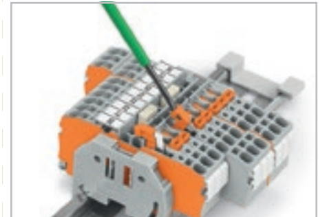
2- и 4-проводные клеммы с размыкателем для тестирования и измерений Ножевой размыкатель закрыт.
