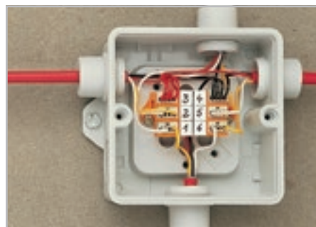
Типовое применение в клемме для охранной сигнализации – винтовое крепление
