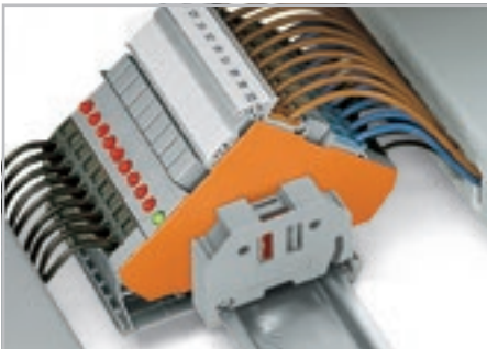
Клеммы для датчиков. Подача питания со стороны датчика
