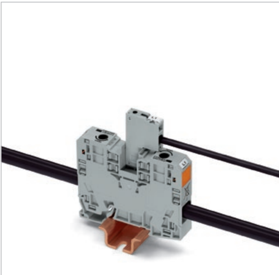
Боковое подключение означает, что даже большие проводники с ограниченной гибкостью могут быть легко подключены.
