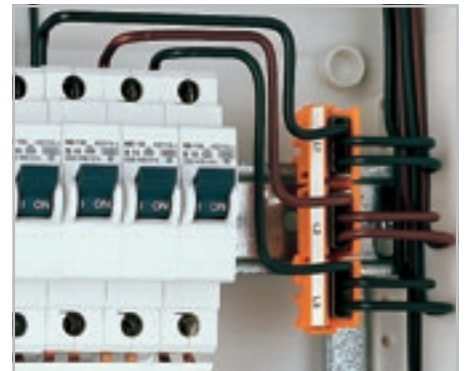
ЗАФИКСИРОВАННОЕ ПОЛОЖЕНИЕ - на DIN-рейке 35 мм
