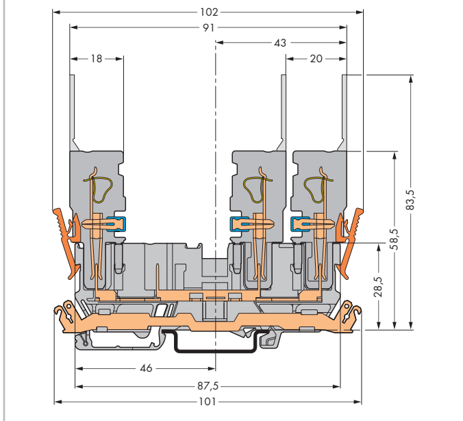
Базовая клемма с экранированным контактом
