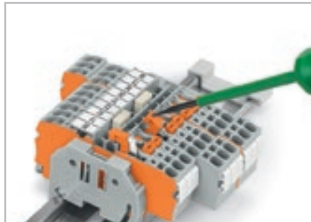
2- и 4-проводные клеммы с размыкателем для тестирования и измерений Ножевой размыкатель открыт.
