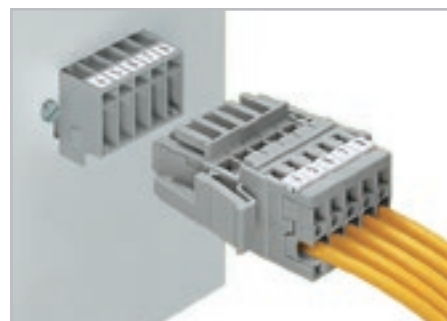
Вилка с крепежными фланцами и 1-проводная розетка с боковым фиксирующим рычагом
