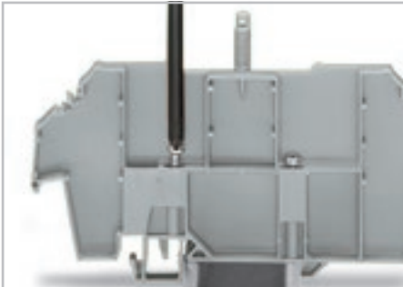
Затяните зажимной винт (слева) и крепежный винт (справа).
