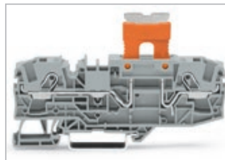
Базовая клемма с размыкателем в исходном положении.
