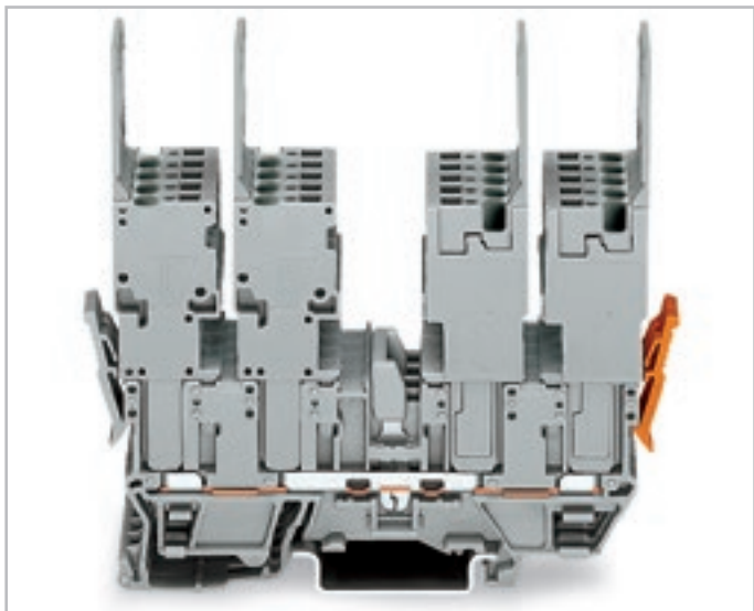
4 x 1-проводная розетка – Объединение базовых клемм с помощью перемычек серии 280 и 780, проверка с помощью тестового адаптера 280-404.
