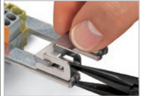
Для извлечения шины сожмите пружину с помощью плоскогубцев.
