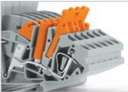
Перемычка с предохранительным колпачком - Перемычка с поднятым предохранительным колпачком
