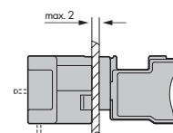
Штекер-розетка с боковым фиксирующим рычагом
