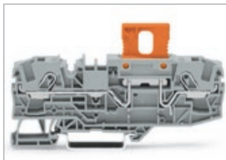
Базовая клемма с размыкателем в рабочем положении.
