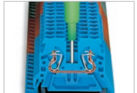
Тестирование с помощью прибора для замера фазы, так же возможно использование одноконтактного индикатора напряжения.
