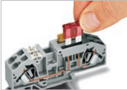
Установка предохранителя
