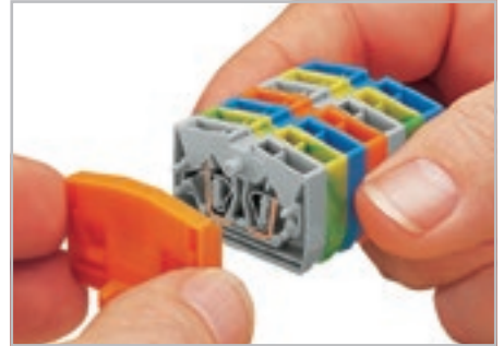
Установка торцевой пластины.
