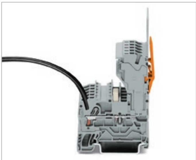
1-проводная розетка Объединение базовых клемм возможно с помощью гребешковых перемычек серии 2002.
