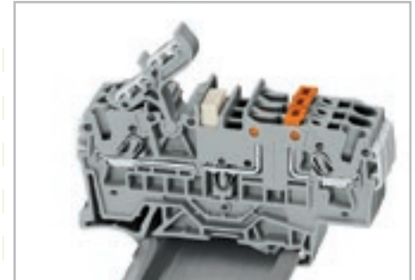
Дополнительная возможность маркировки с поворотным маркировочным адаптером
