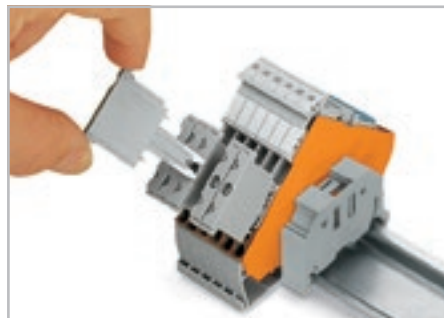
Клеммы для исполнительных устройств с штекерами для компонентов (280-801).
