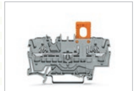
Базовая клемма с размыкателем в рабочем положении.
