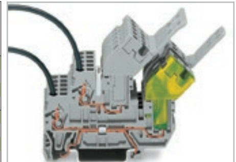
Розетки углового исполнения обеспечивают уменьшение высоты установки
