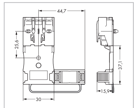
Габаритные размеры в мм
