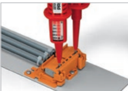
Испытание соединителей при помощи измерит. гнезд в верхней части держателя.
