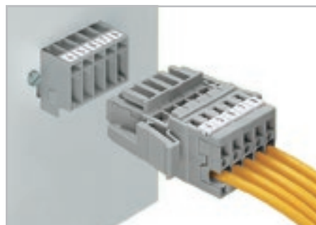
Штекер с прямыми или угловыми выводами под пайку и фиксированными фланцами 1-проводная прямая розетка с поперечными фиксирующими рычагами
