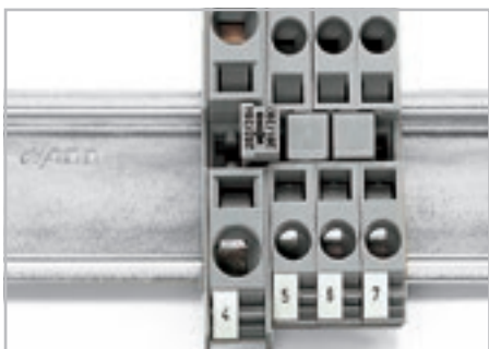
Примечание: перемычки, маркированы подходящими размерами клемм для правильной установки.
