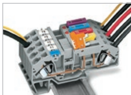
Питание через размыкатель. Размыкатель для всех контактов объединенных клемм с предохранителями.
