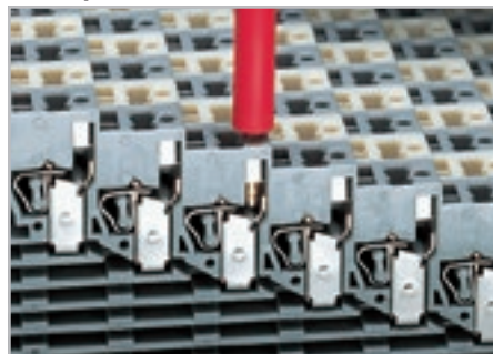
Специальный тестовый контакт для тестового штекера 2,3 мм Ø.
