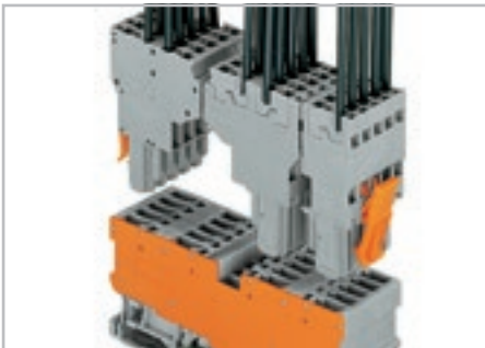
4-контактная базовая клемма 2-проводная розетка 1-проводная розетка, прямая
