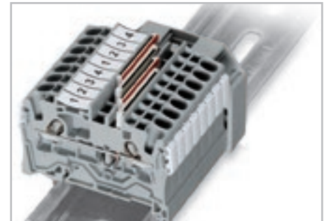
Разместите красные полосы ступенчатых перемычек изнутри
