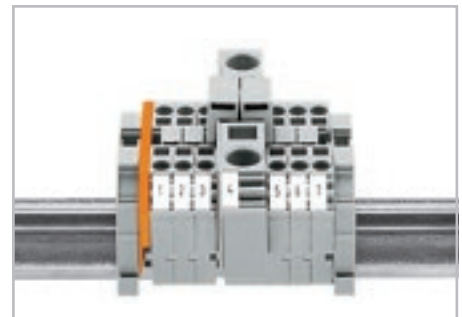
Объединение клемм от 16 мм 2 /AWG 6 (серия 283) до 4 мм 2 /AWG 12 (серия 281) для монтажа на рейку.
