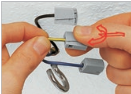
Отключение: удерживая проводник и прокручивая его вправо-влево, извлечь проводник.
