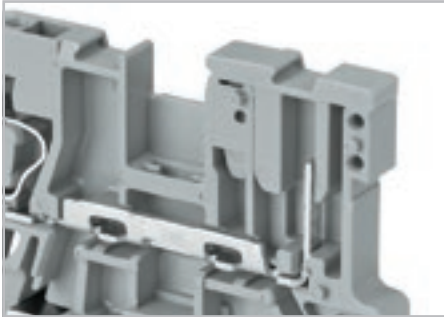
Крышка вывода с держателем для mini-WSB
